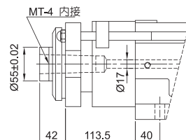
SWD8-150-MT4
