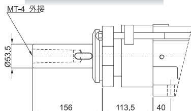
SWD8-150-MT4A
